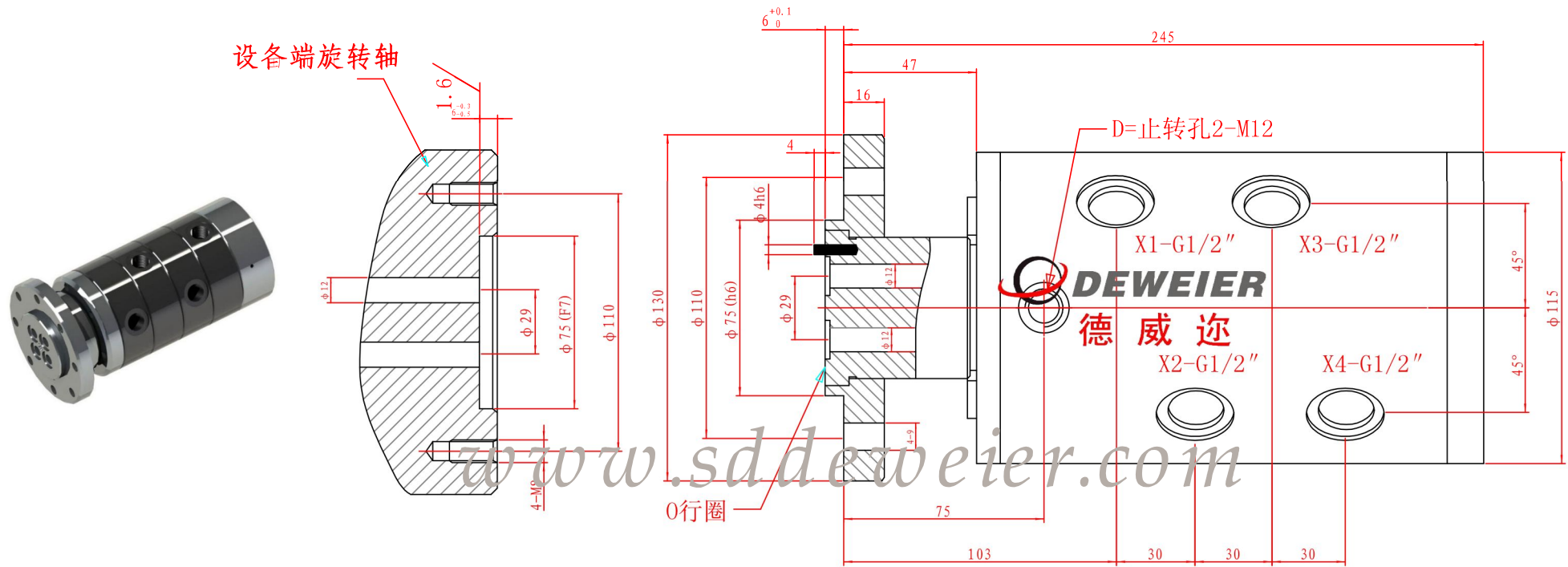
液压四通道旋转接头-DRF04015
