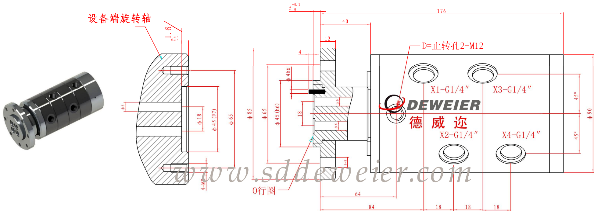
液压四通道旋转接头-DRF04008
