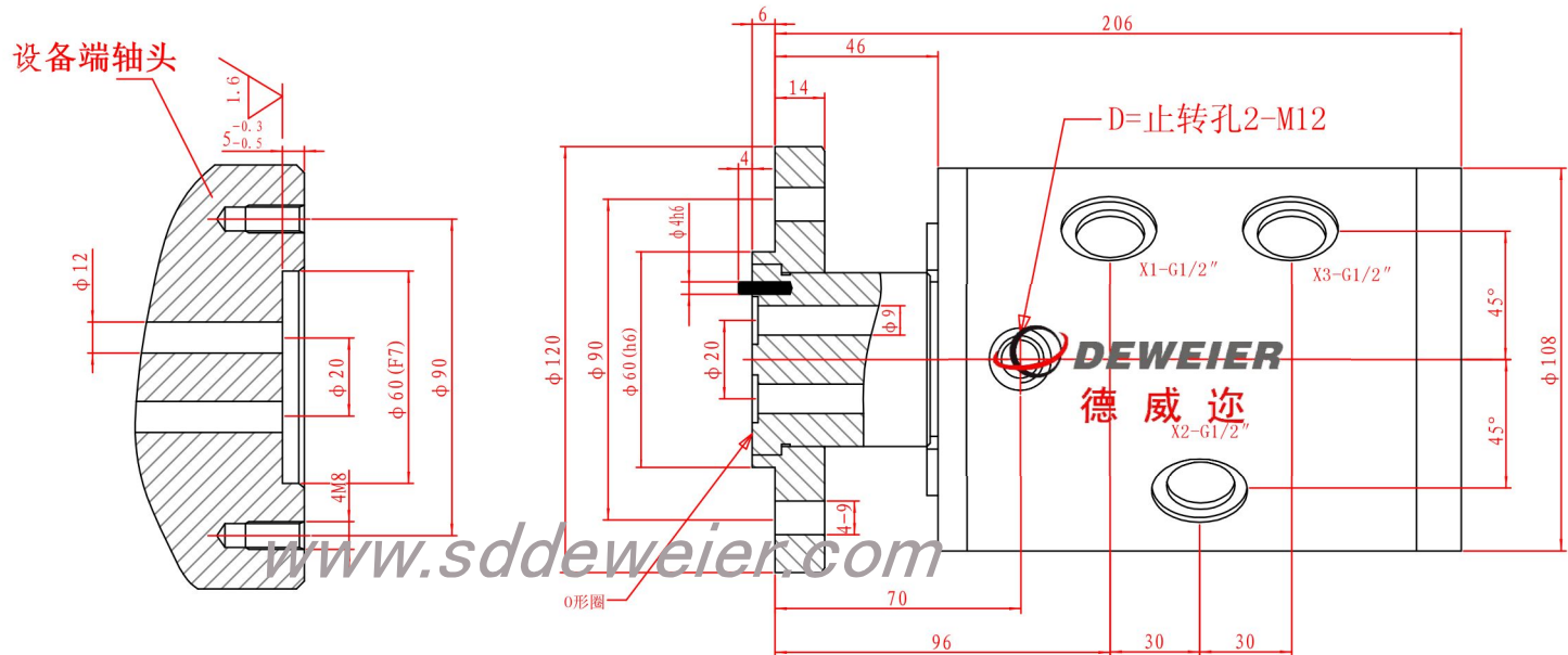
液压三通道旋转接头-DRF03015
